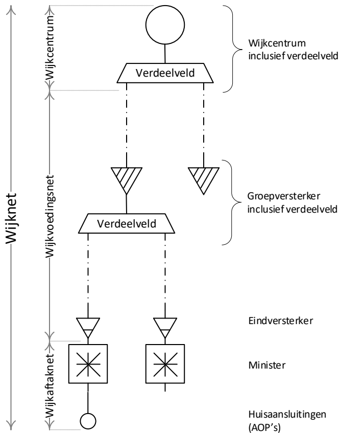
5-1 Standaard wijknetconcept
